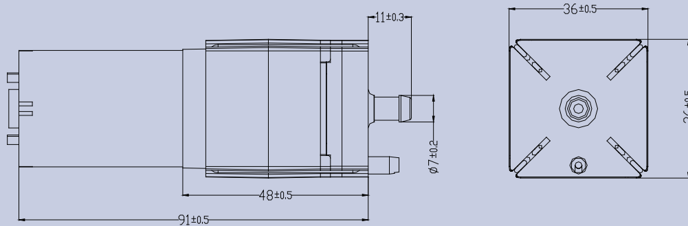
產品構造圖 Dimension Drawing
