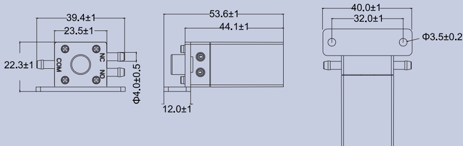
產品構造圖 Dimension Drawing
