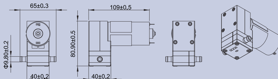
產品構造圖 Dimension Drawing
