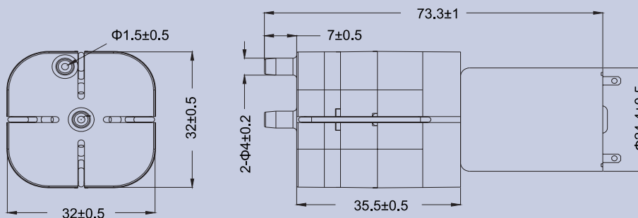
產品構造圖 Dimension Drawing
