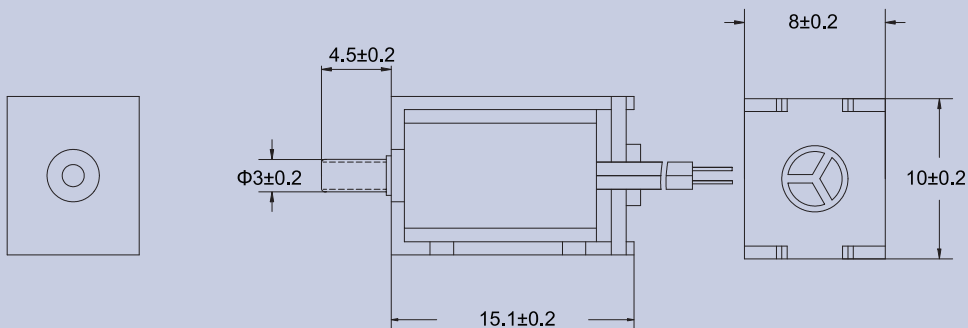
產品構造圖 Dimension Drawing
