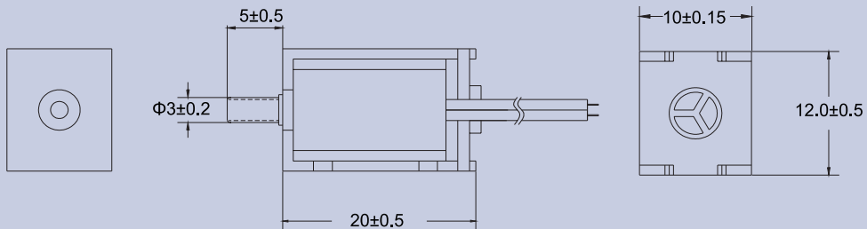
產品構造圖 Dimension Drawing
