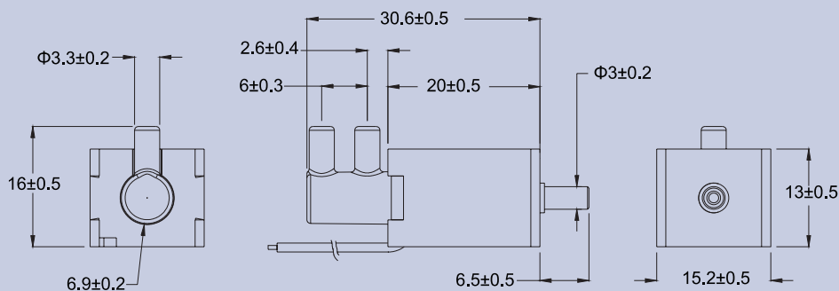
產品構造圖 Dimension Drawing
