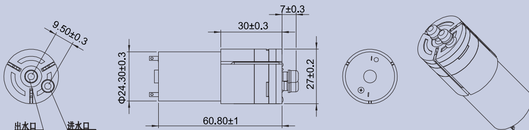
產品構造圖 Dimension Drawing
