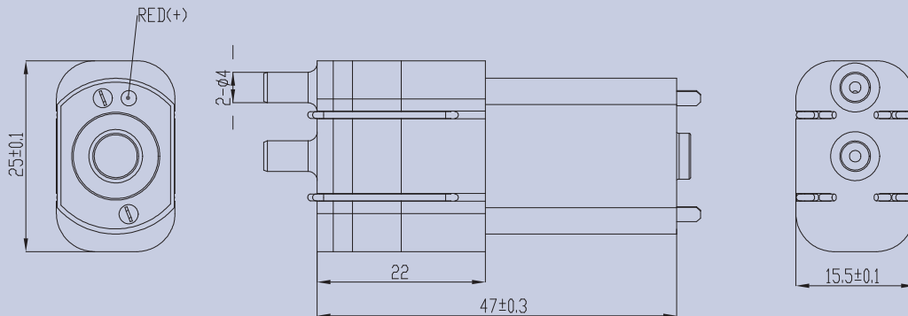
產品構造圖 Dimension Drawing
