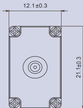
產品構造圖 Dimension Drawing
