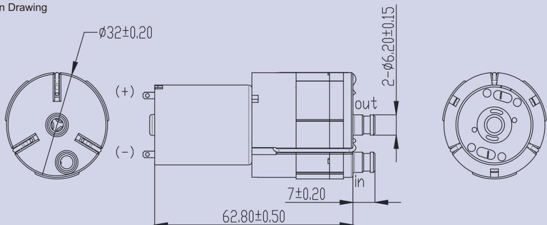
產品構造圖 Dimension Drawing
