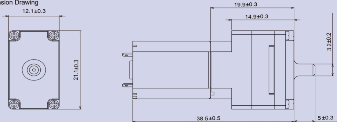
產品構造圖 Dimension Drawing
