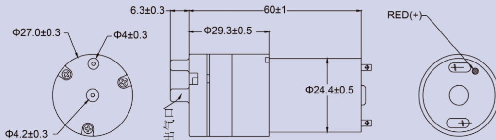
產品構造圖 Dimension Drawing
