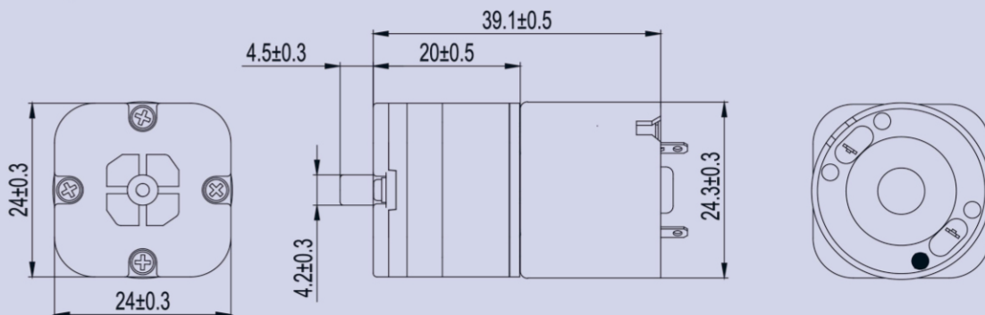
產品構造圖 Dimension Drawing
