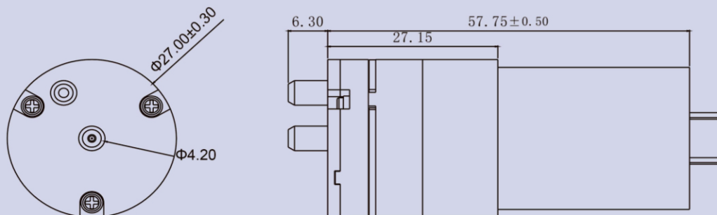
產品構造圖 Dimension Drawing
