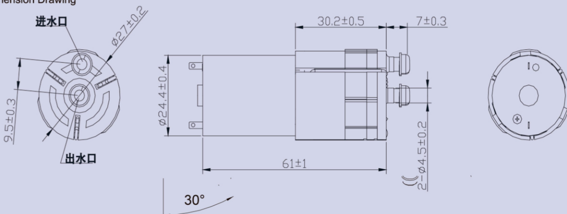
產品構造圖 Dimension Drawing
